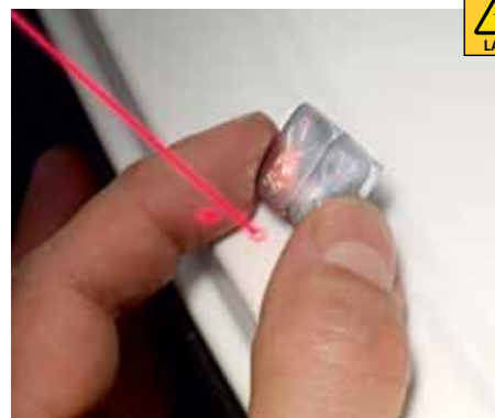
Punkt laser zur präzisen Positionierung der Klebgewichte an Alufelgen (innen und hinter den Speichen)
