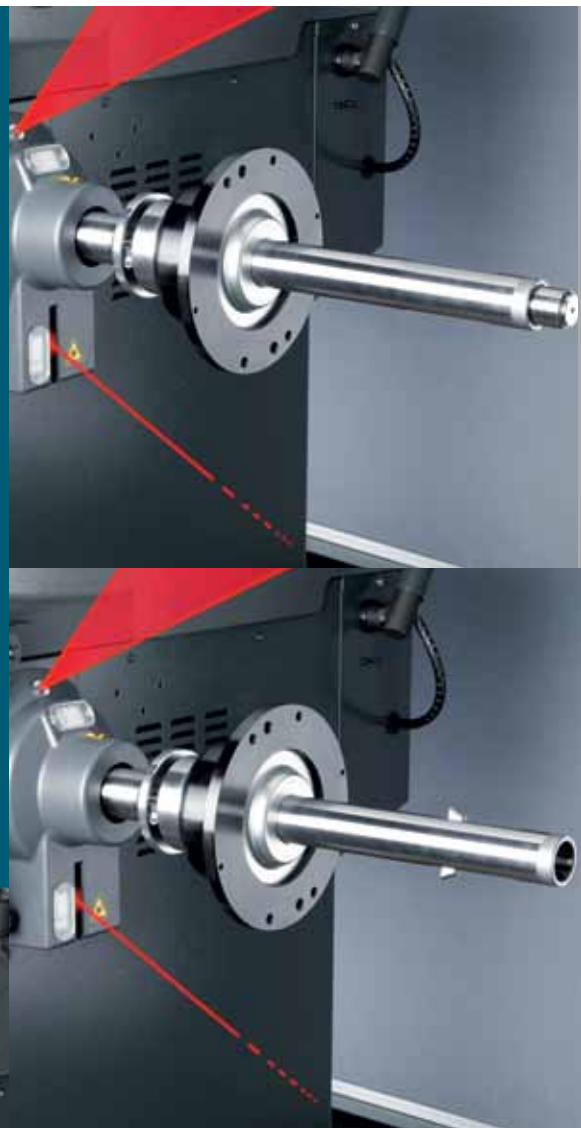
Pneumatischer Flansch: Einfach ... schnell ... fest.
